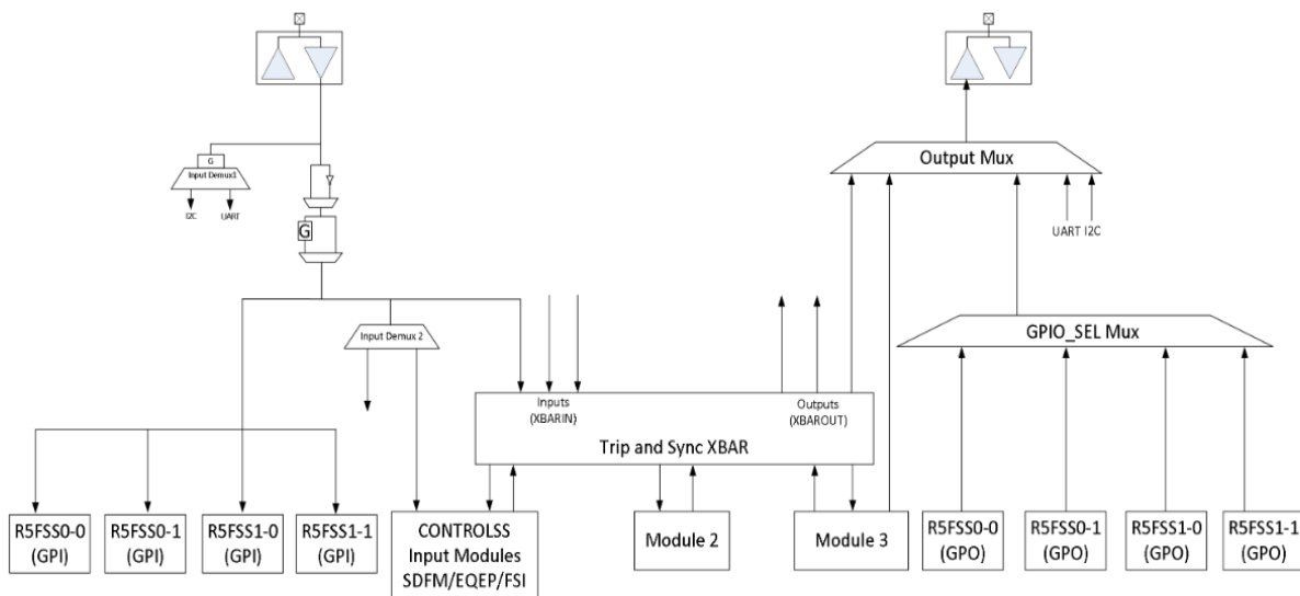
Slika 7. Shema GPIO te multiplesor i XBAR modula i njihova međusobna povezanost [31]
