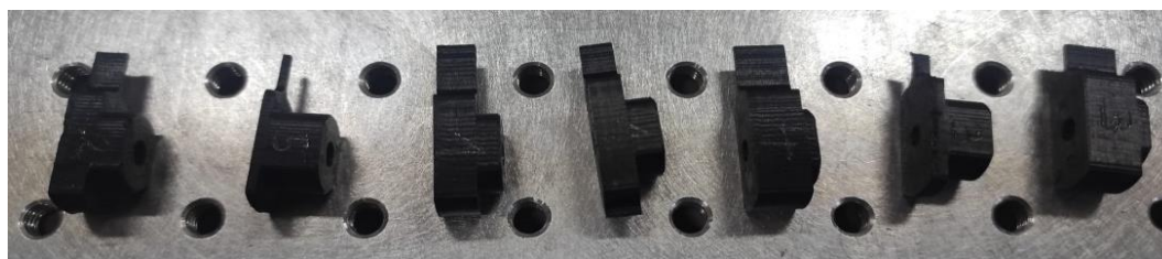
Slika 5.5 Prikaz 3D tiskanih rotora s različitom geometrijom trzalica
