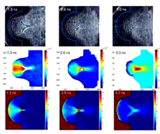
Slika 3.4. Hologramski snimak
