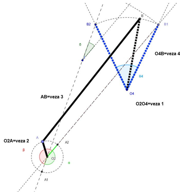
Slika 16 Četveročlani brospovratni mehanizam
