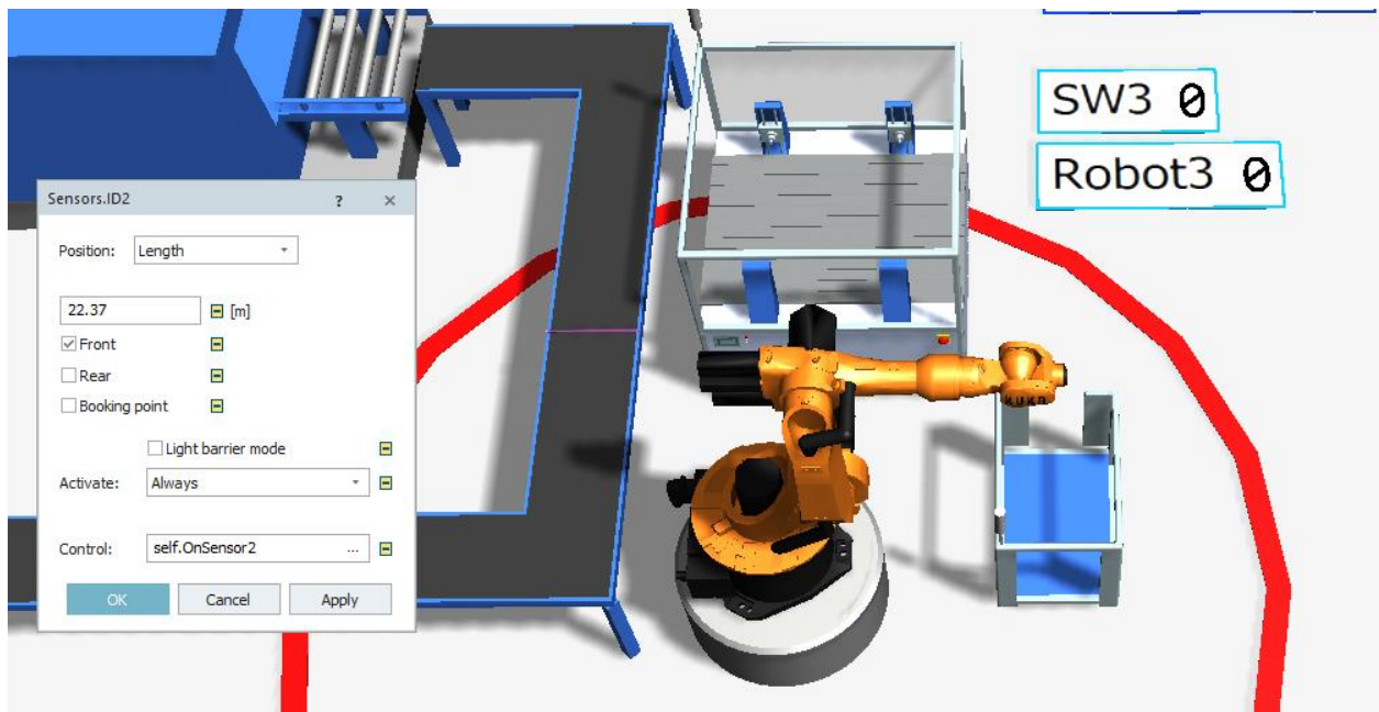
Slika 5.29 Prvi senzor na velikoj pokretnoj traci
