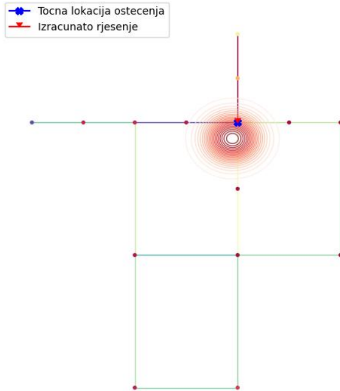
Slika 6.2 Prikaz rješanja i pretpostavke modela – slučaj 1
