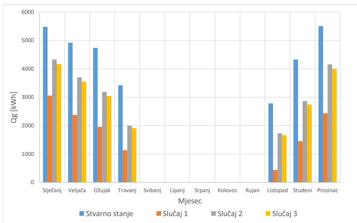
Slika 3.3. Ukupna potreba za toplineom kroz cijelu godinu
