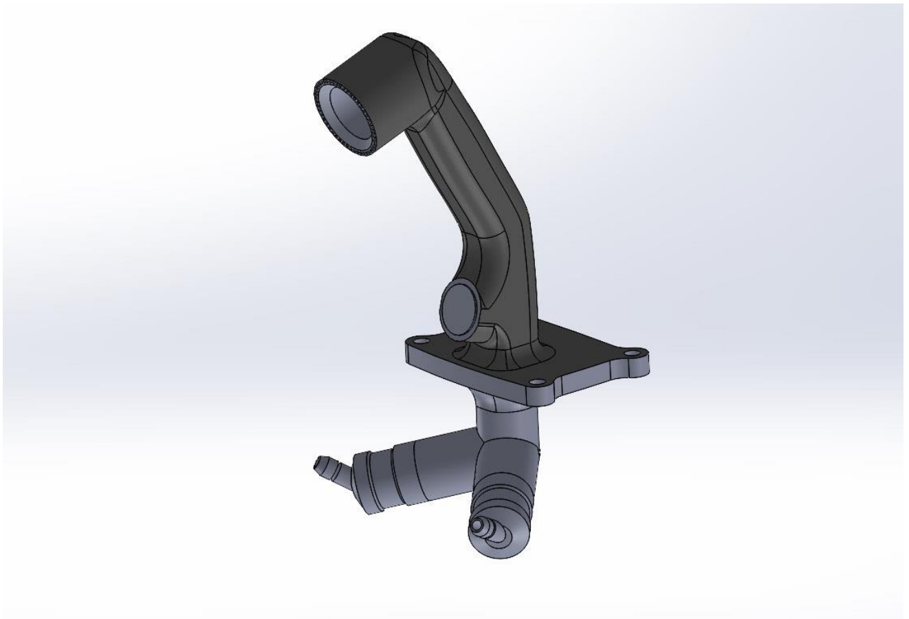
Slika 25 3D model mlaznice za gorivo
