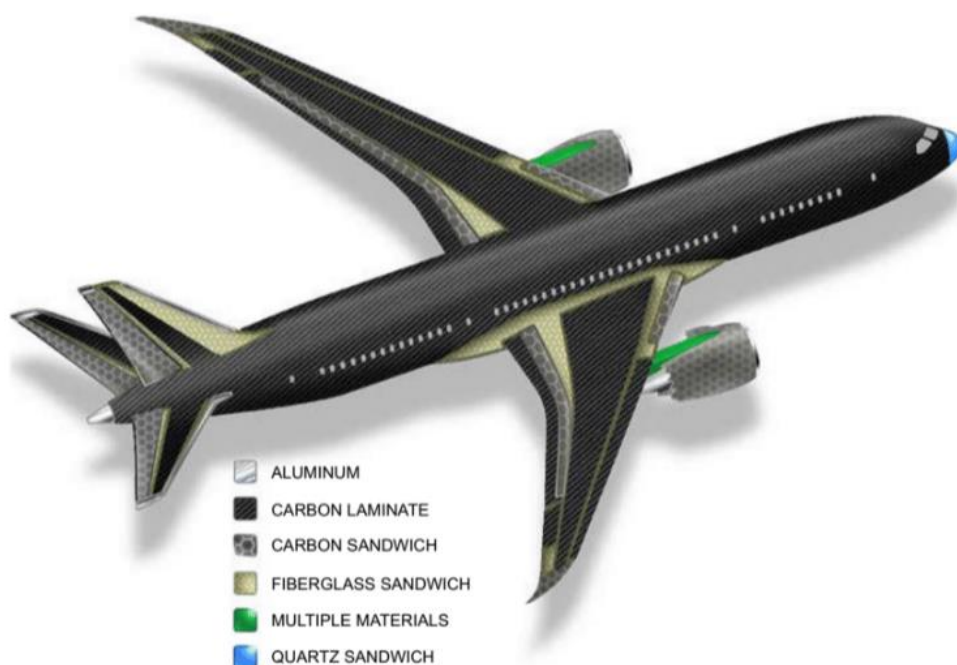
Slika 18 Struktura Boeinga 787 [3]
