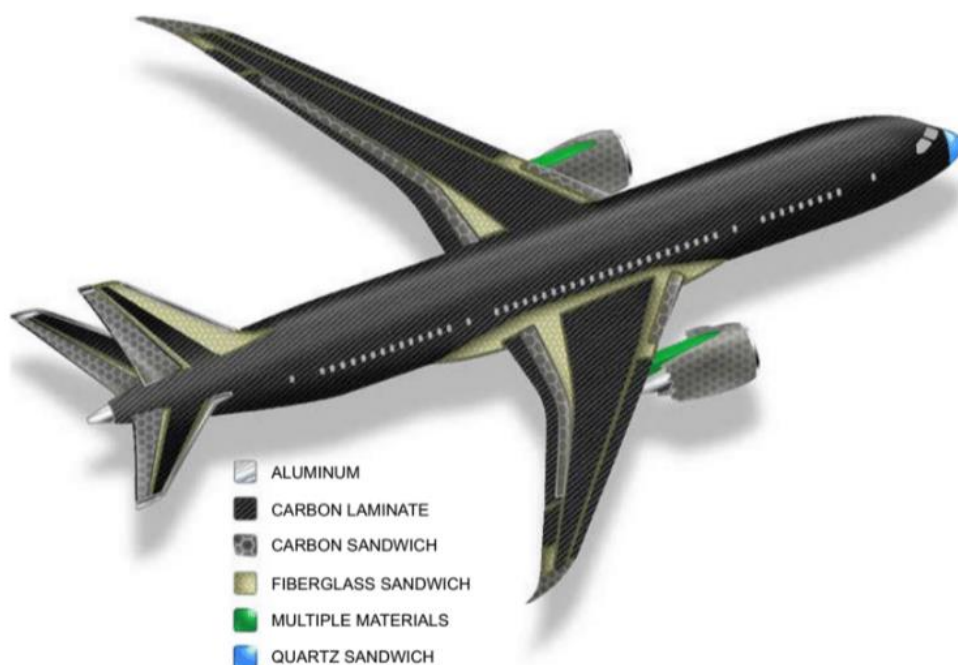
Slika 18 Struktura Boeinga 787 [3]
