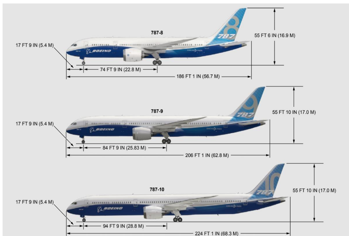
Slika 17 Usporedba Boeinga 787-8/9/10 [3]
