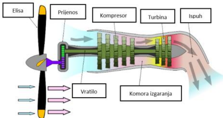
Slika 5 Turbo-propelerni motor [2]
