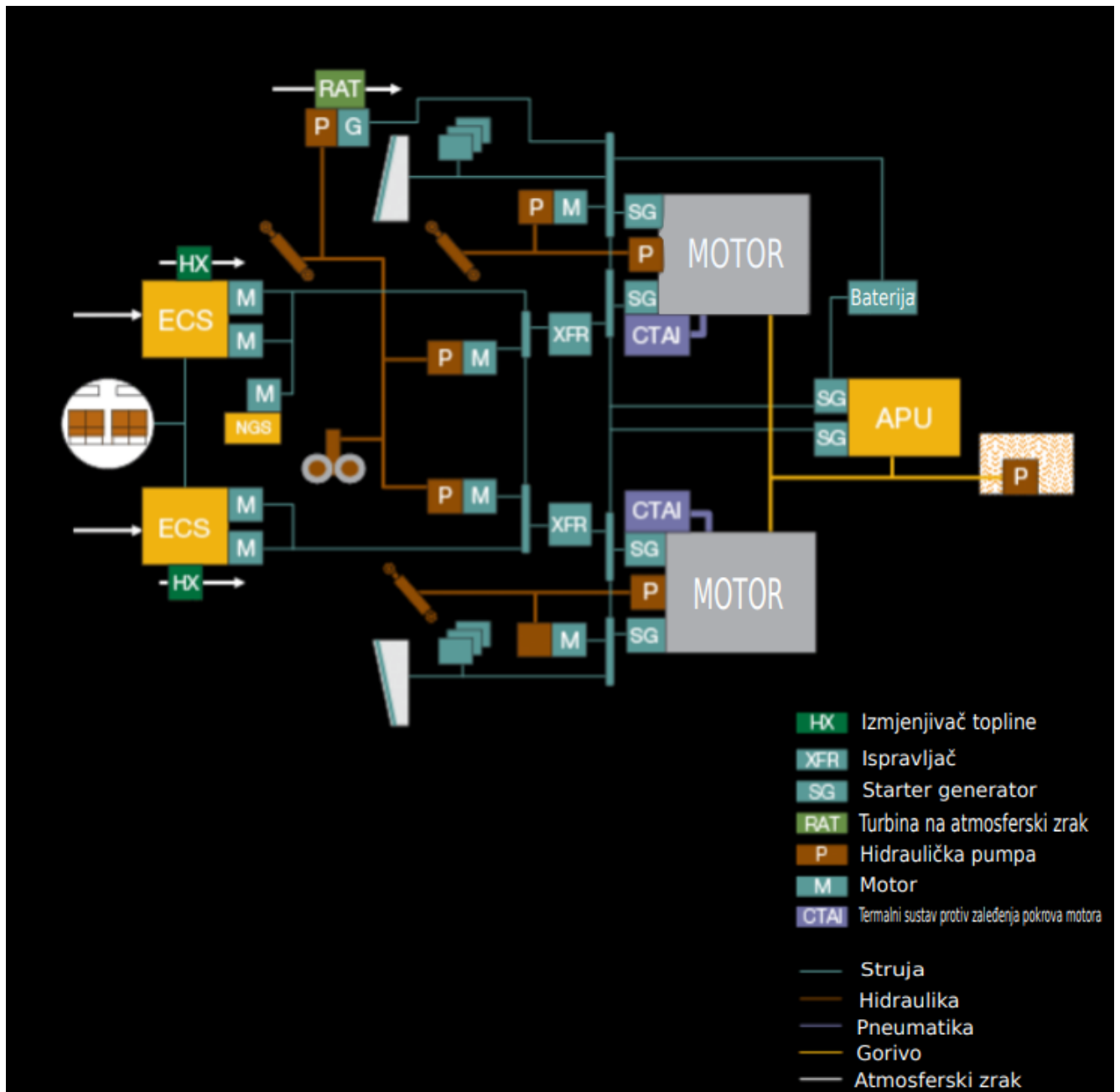
Slika 23 Elektro-shema Boeinga 787
