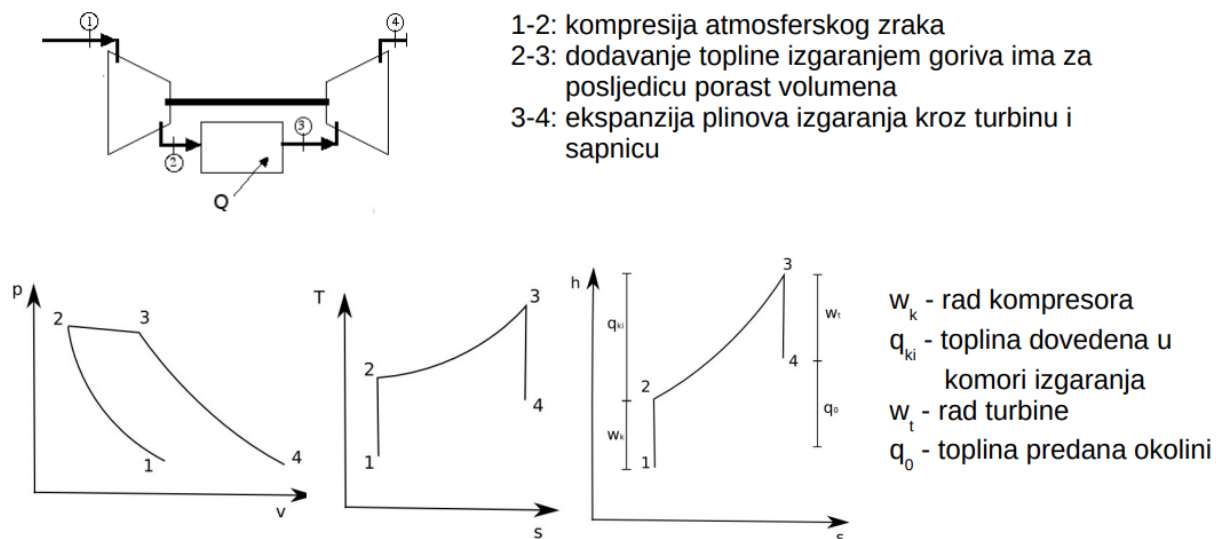
Slika 2 Princip rada mlaznih motora [2]
