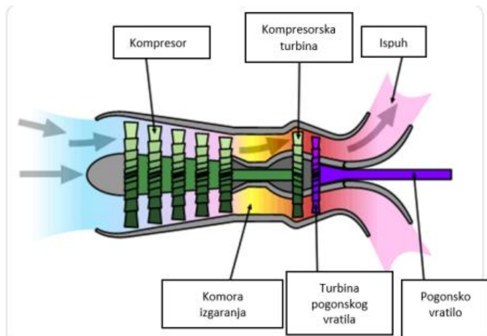
Slika 6 Turbo-osovinski motor [2]
