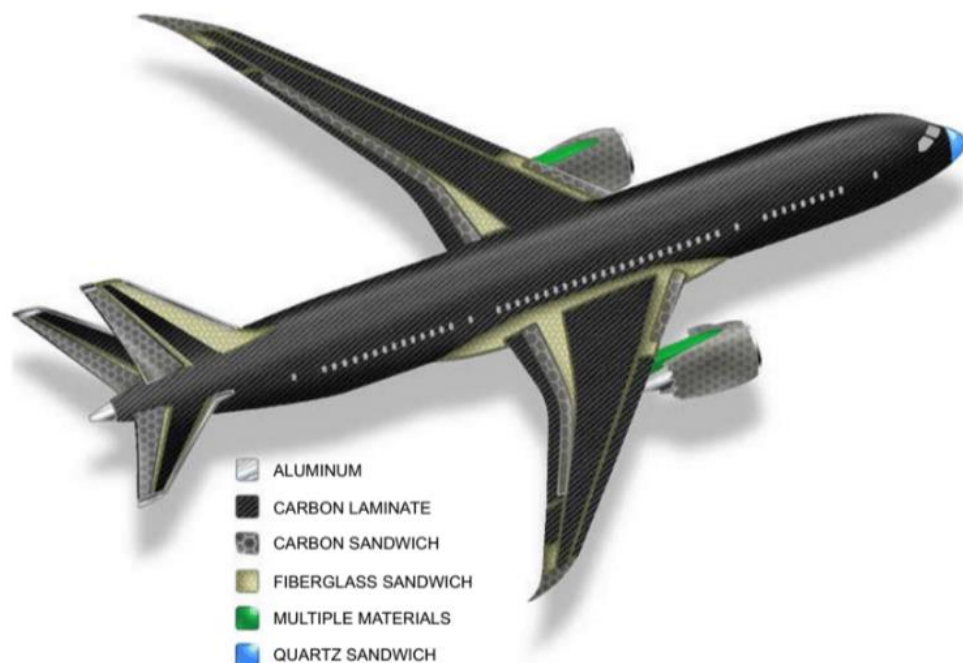
Slika 18 Struktura Boeinga 787 [3]
