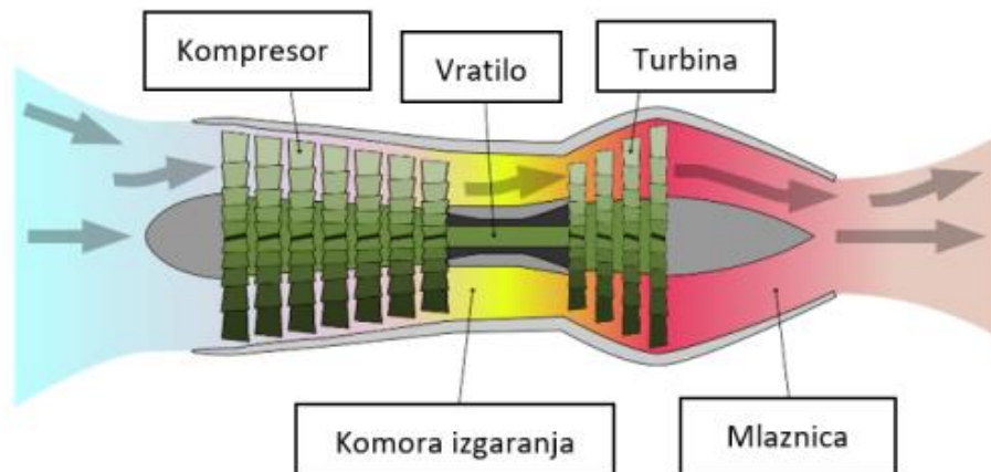
Slika 3 Turbo-mlazni motor [2]
