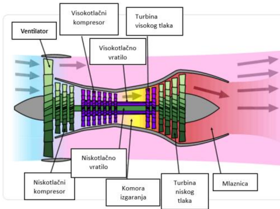
Slika 4 Turbo-ventilatorski motor [2]
