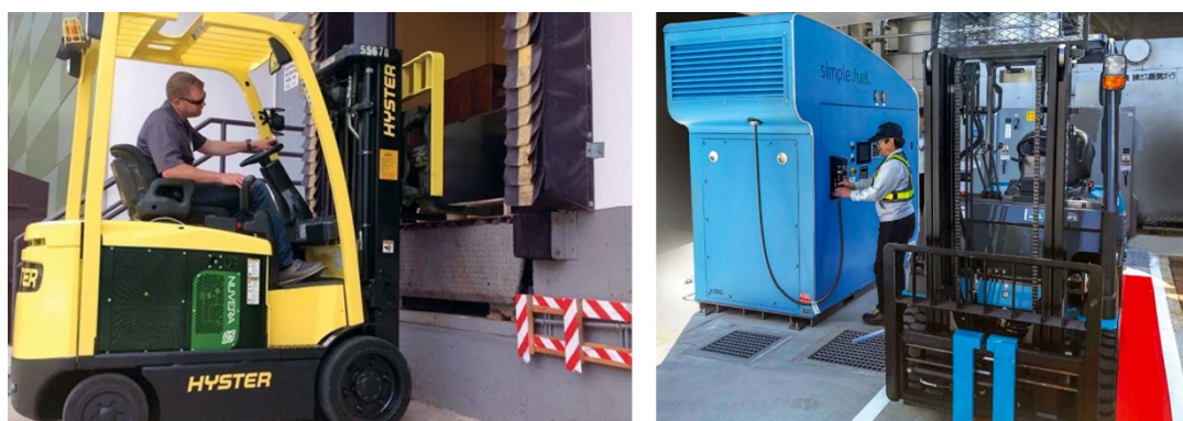
Slika 4.10 Viličar na vodik grupe Hyster; punjenje viličara vodikom. [25]
