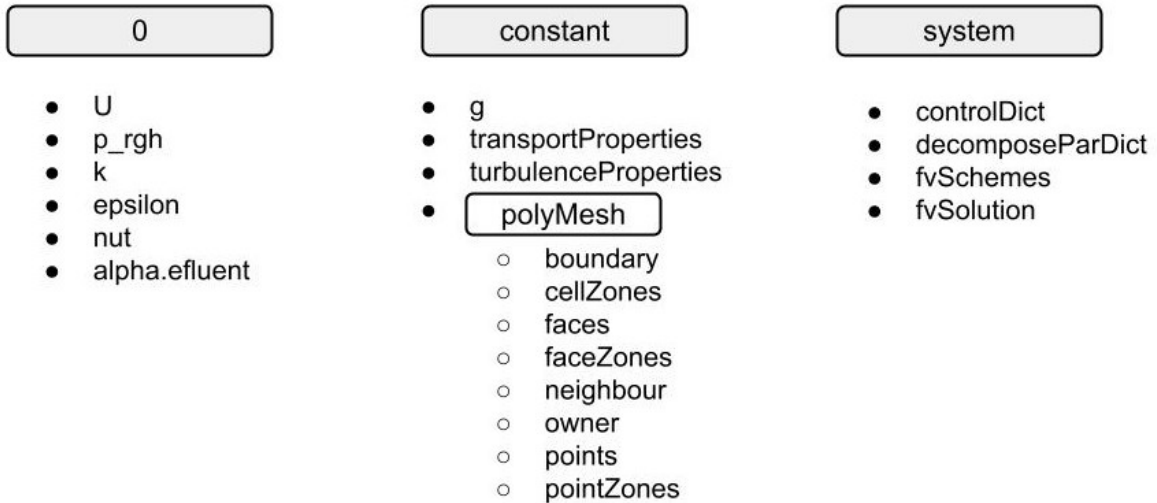
Slika 2.3: Struktura OpenFOAM modela te prikaz podmapa i datoteka
