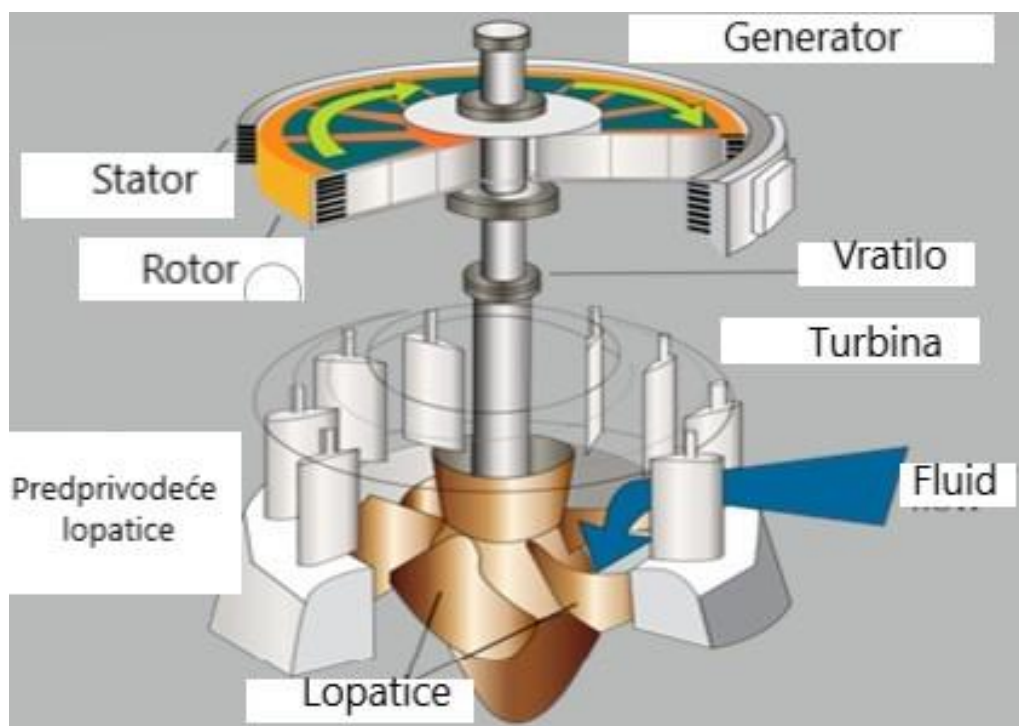
Slika 3.1 Prikaz Kaplanove turbine s generatorom [6]
