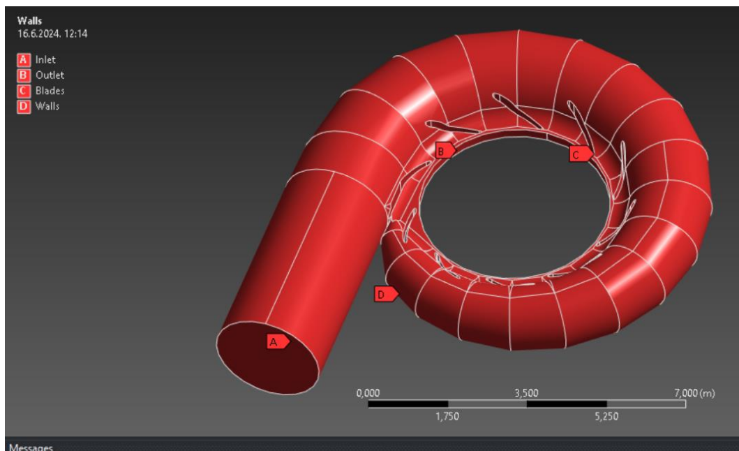
Slika 5.13 Rubni uvjeti
