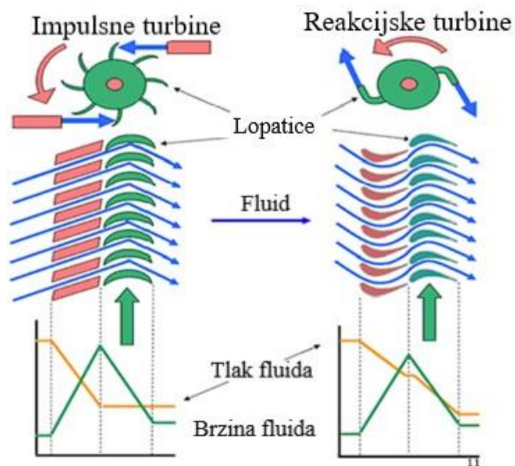
Slika 2.1 Razlika između akcijske i reakcijske turbine [2]
