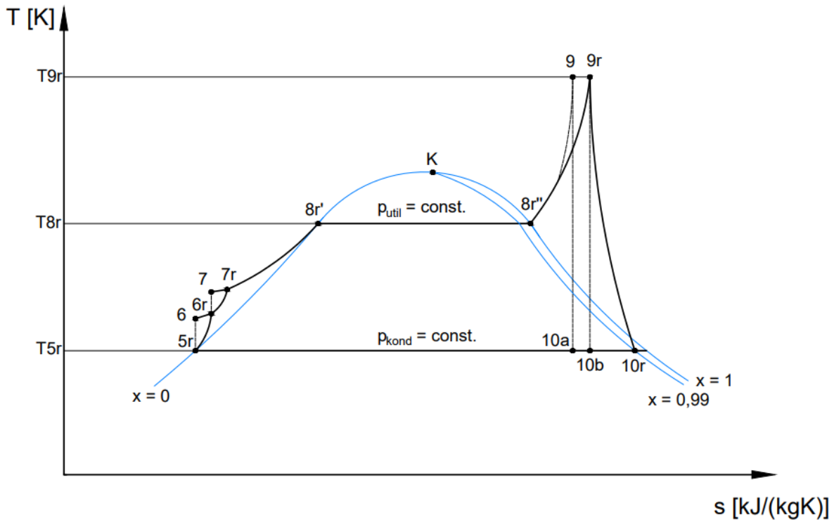
Slika 3.5. T-s dijagram parnog dijela procesa
