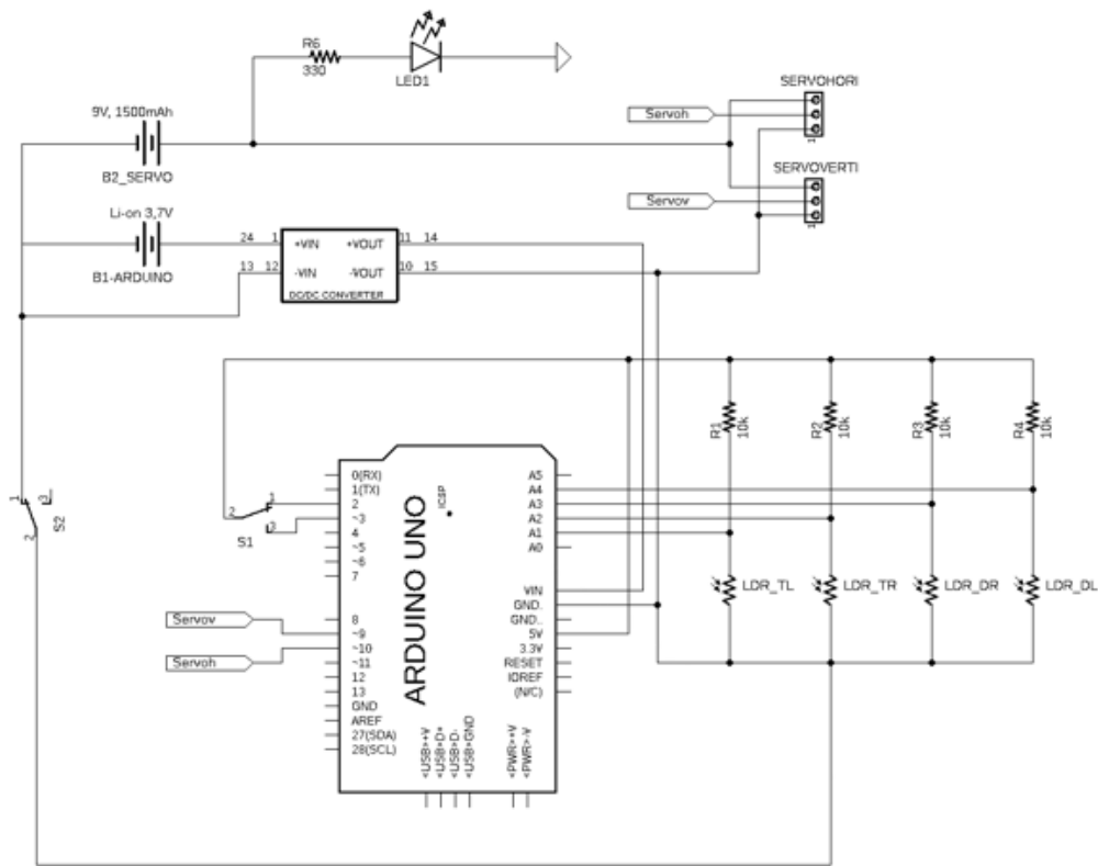
Slika 9.1. Shema spoja.
