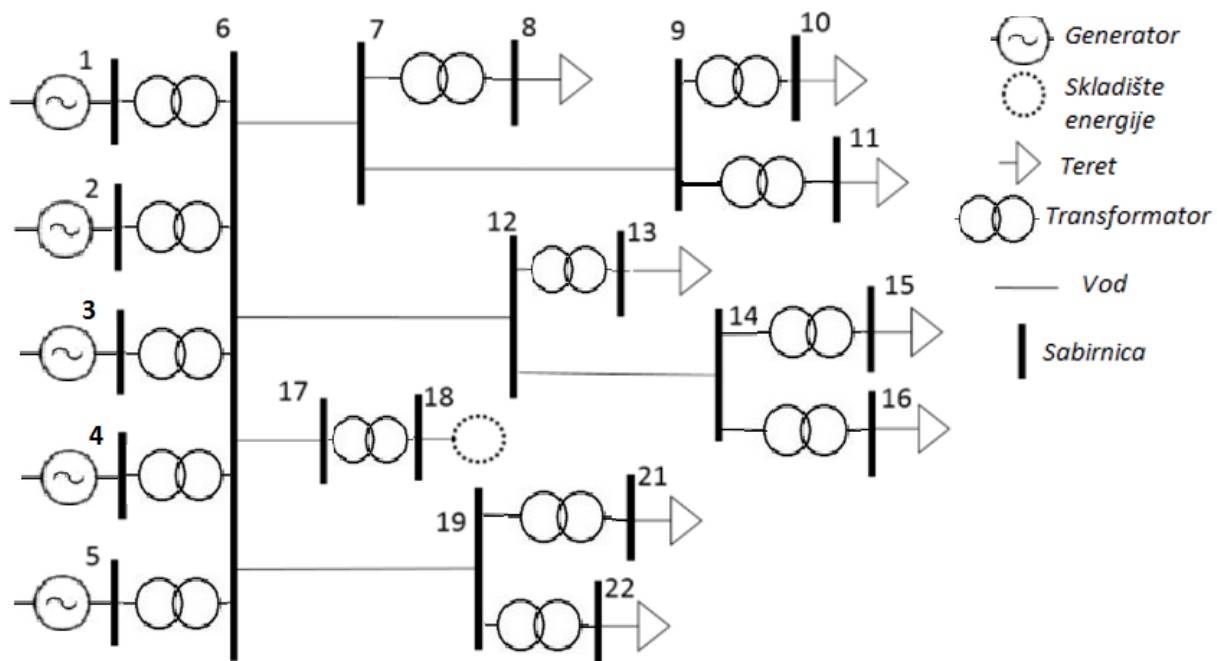
Slika 5.4. Otočni sustav [1]
