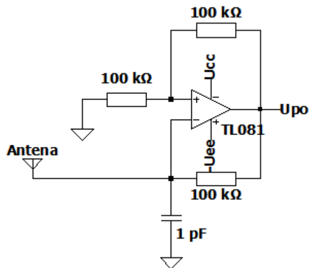
Slika 11. Promjenjivi oscilator visine tona (LTspice)
