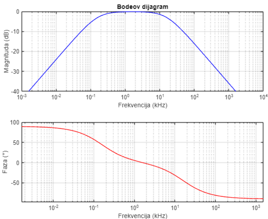
Slika 14. Bodeov dijagram pojavnog filtera
