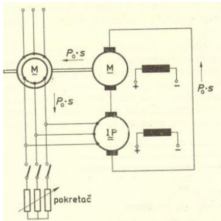
Slika 9.1 Krämerova kaskada
