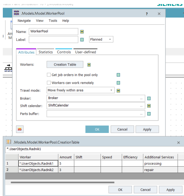
Slika 4.35 - Postavke WorkerPool-a
