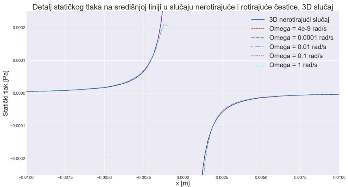
Slika 6.21 Detalj statičkog tlaka na središnjoj liniji
