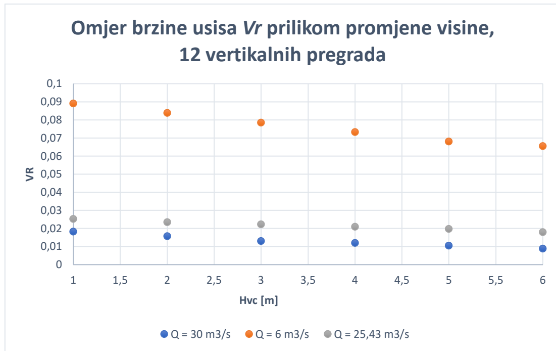
Slika 7.27 Omjer brzine Vr prilikom promjene visine 12 pregrada
