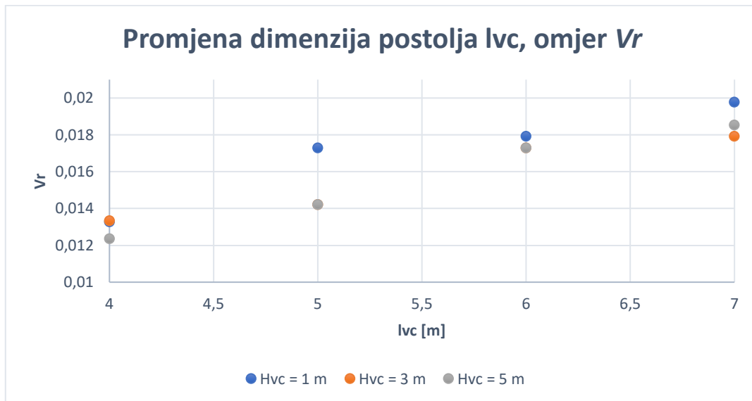
Slika 7.35 Promjena dimenzija postolja l_{vc} - omjer brzine usisa V_r
