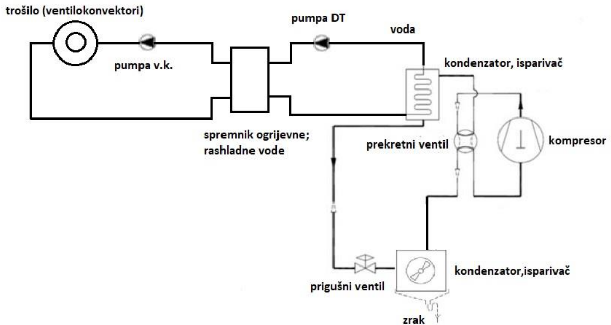
Slika 8.3 Pojednostavljena shema sustava grijanja i hlađenja DT zrak – voda
