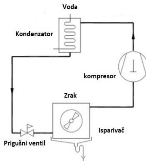
Slika 8.2 Shema dizalice topline zrak – voda [8]
