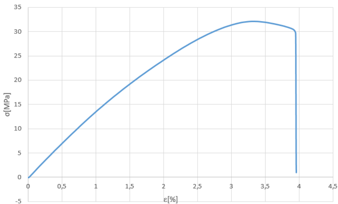
\sigma - \epsilon dijagram (ABS bazni uzorak- serija 2)
