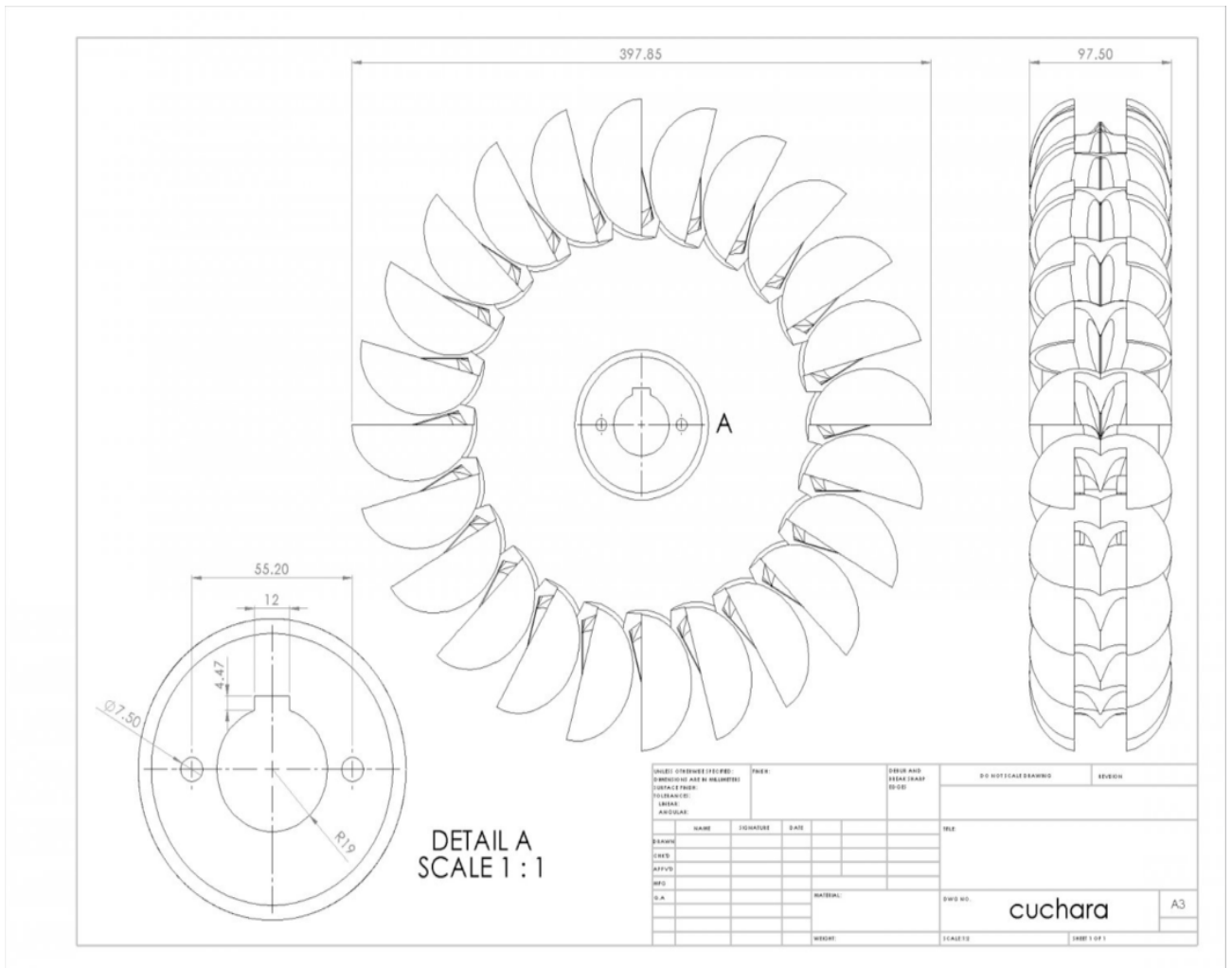
Slika 5.1. Nacrt turbine tvrtke 3DEXPORT [3]
