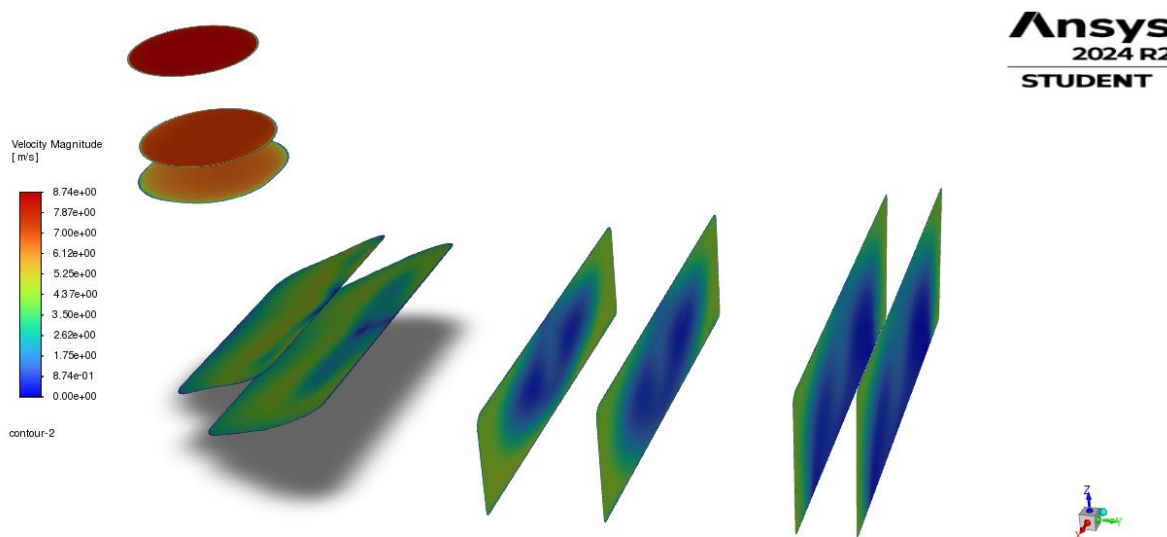
Slika 8.10 Prikaz kontura brzine u difuzoru presjeka YZ ravninom
