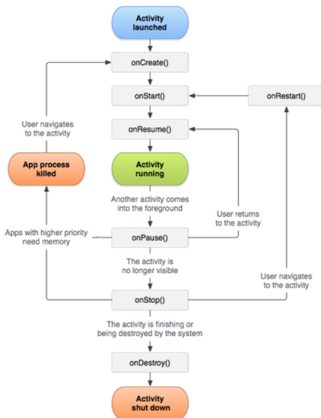
Slika 4.1 Pojednostavljeni prikaz životnog ciklusa aktivnosti unutar Android Studio razvojnog okruženja za nativne Android aplikacije. [5]
