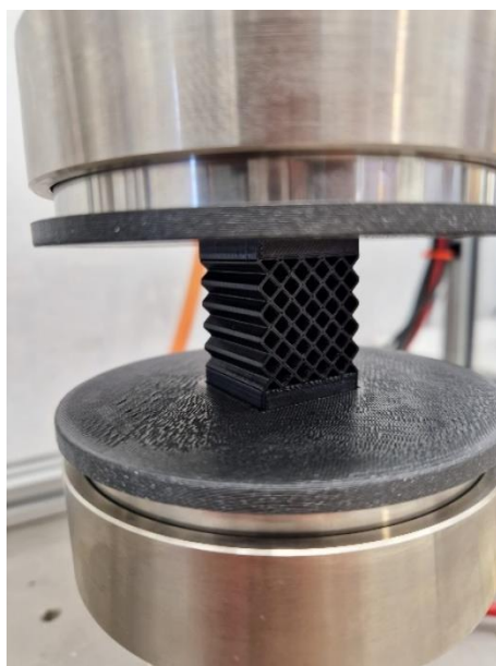
Slika 7: Uzorak PETG prije testiranja
