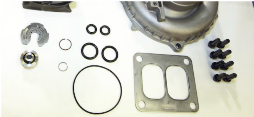
Slica 6.4. Brtva i ležaj turbopuhala
