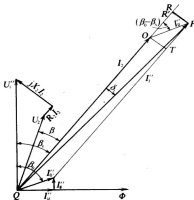
Slika 17: Vektorski dijagram strujnog mjernog transformatora
