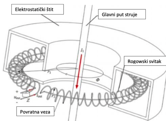
Slika 35: Presjek Rogowskog svitka
