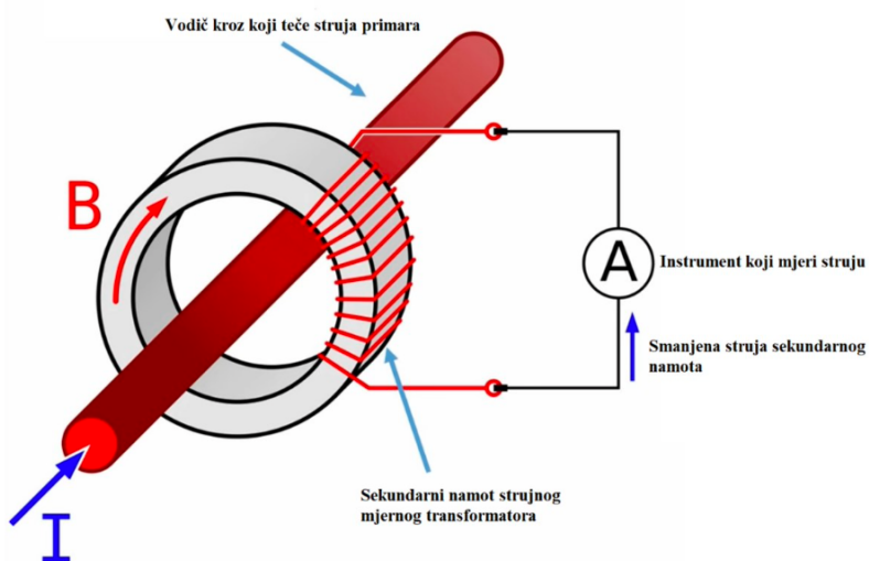
Slika 16: Redukcija i mjerenje struje kroz vodič. [6]
