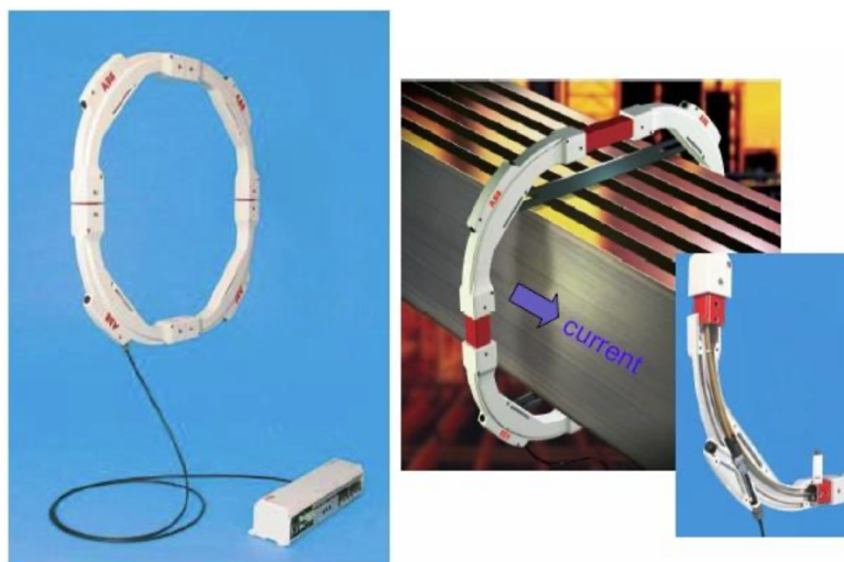
Slika 33: Primjer izvedbe ABB strujnog senzora od optičkih vlakana
