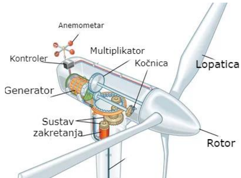
Slika 4.4. Dijelovi turbine
