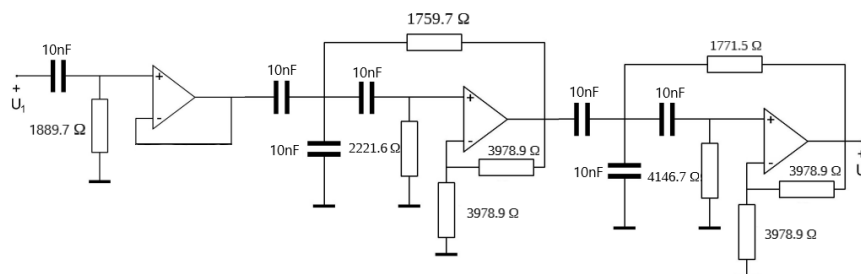
Slika 4.8. Shema VP filtra 5. reda sa denormiranim elementima
