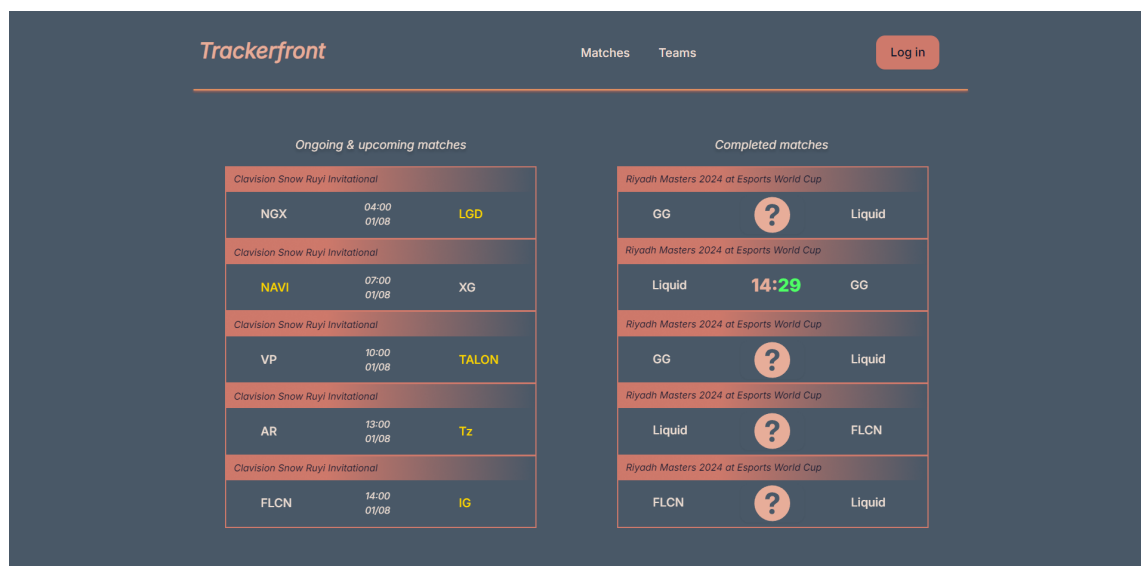
Slika 3.2 Početni prikaz
