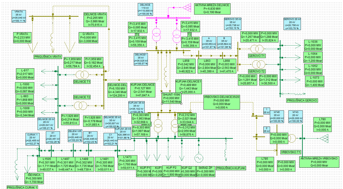
Slika 7.4. Model mreže Gorškog kotara u NEPLAN-u nakon ugradnje prigušnice u TS Delnice
