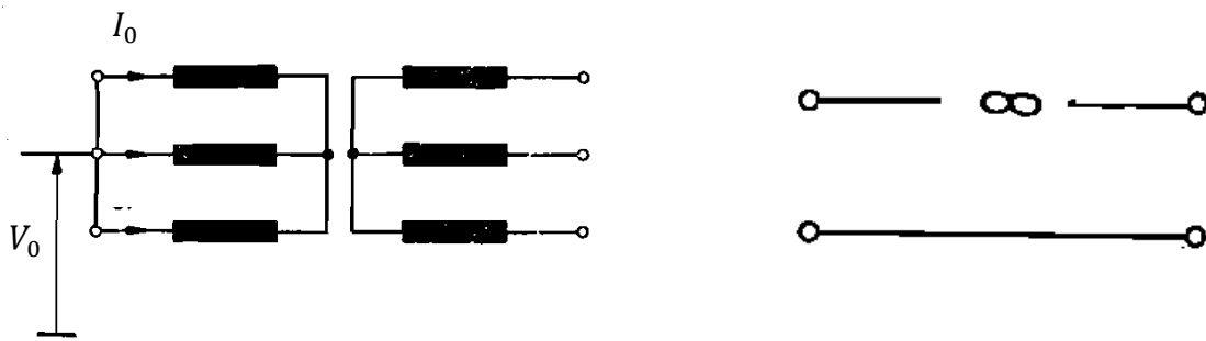
Slika 4.2. Nadomjesna shema spoja zvijezda-zvijezda s izoliranim zvjezditištima [4]
