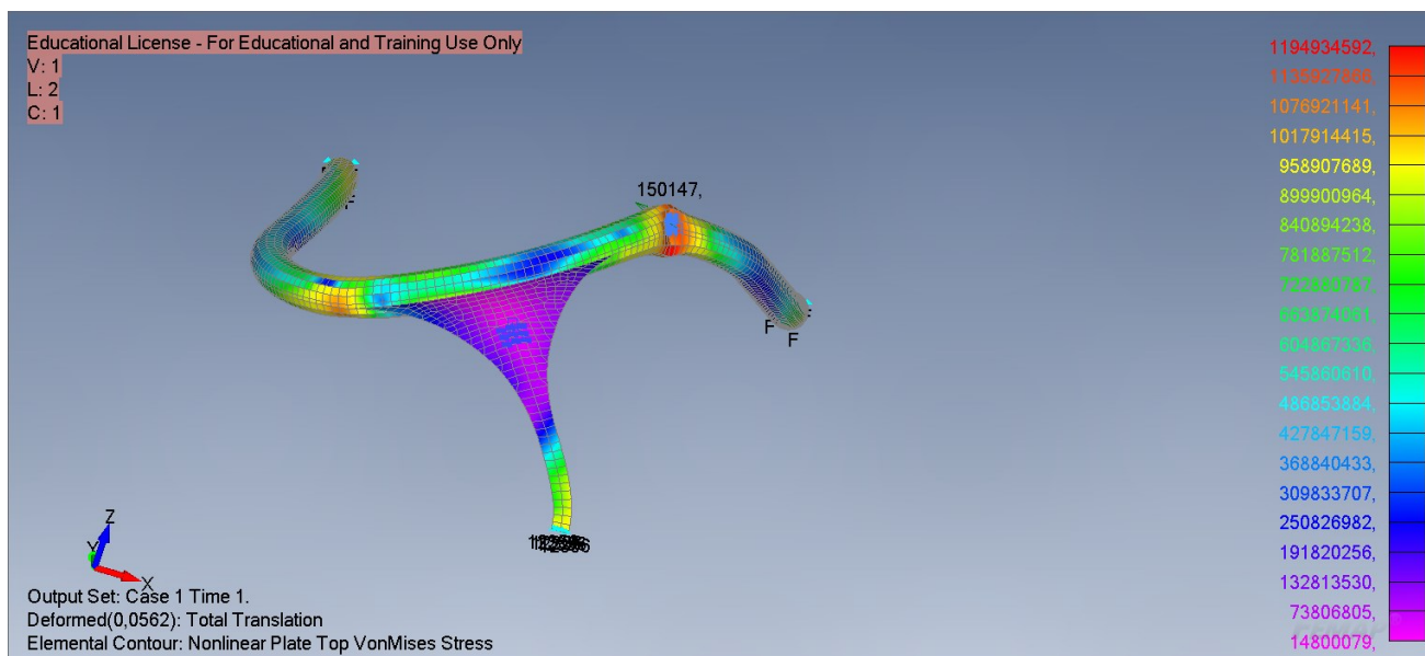
Slika 6.12 Maksimalna naprežanja i deformirani oblik modela s pločastim elementima pod punim opterećenjem, test 2
