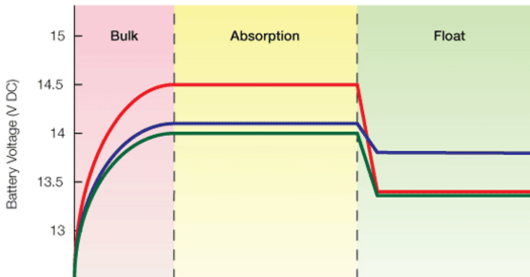
Slika 7.3 3 faze punjenja
