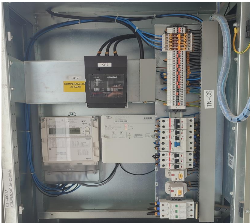
Slika 6.12. Prikaz izgleda mjernog mjesta s ugrađenim sumarnim brojiлом i koncentratorom
