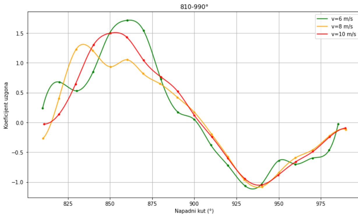
Graf 5.3. Koefficijent uzgona tijekom rotacije pri napadnom kutu 810°-990°
