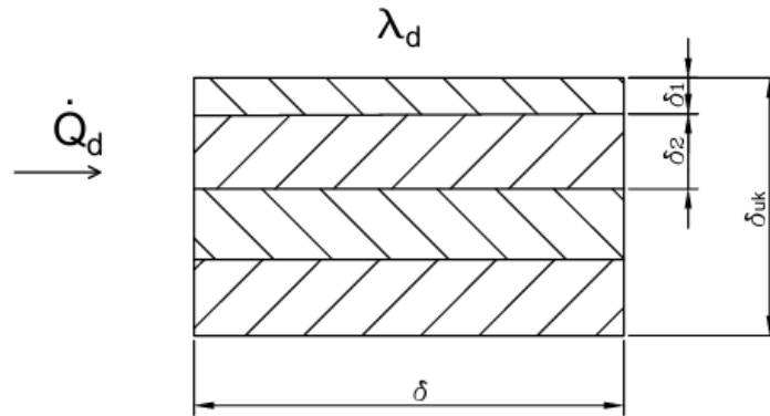
Slika 2.3 Toplinski tok uzduž slojeva stijenske
