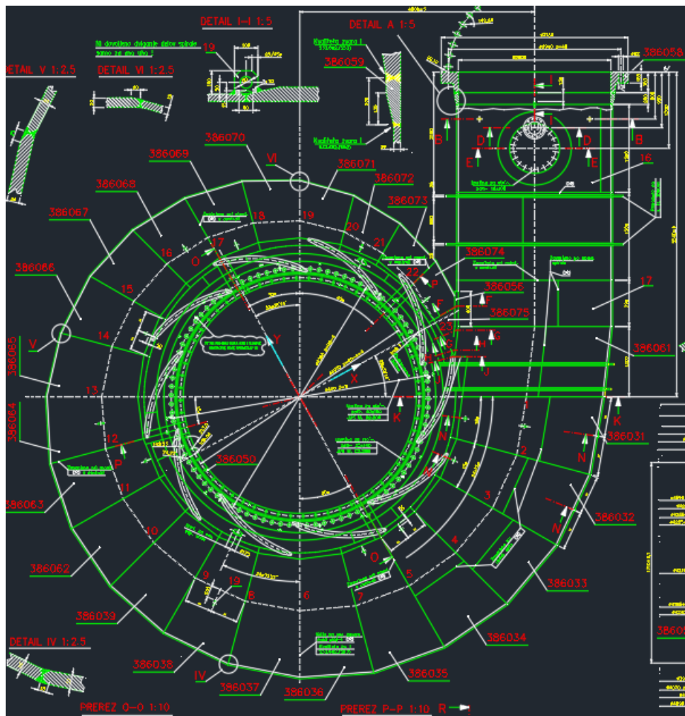
Slika 3-2 Nacrt spirale
