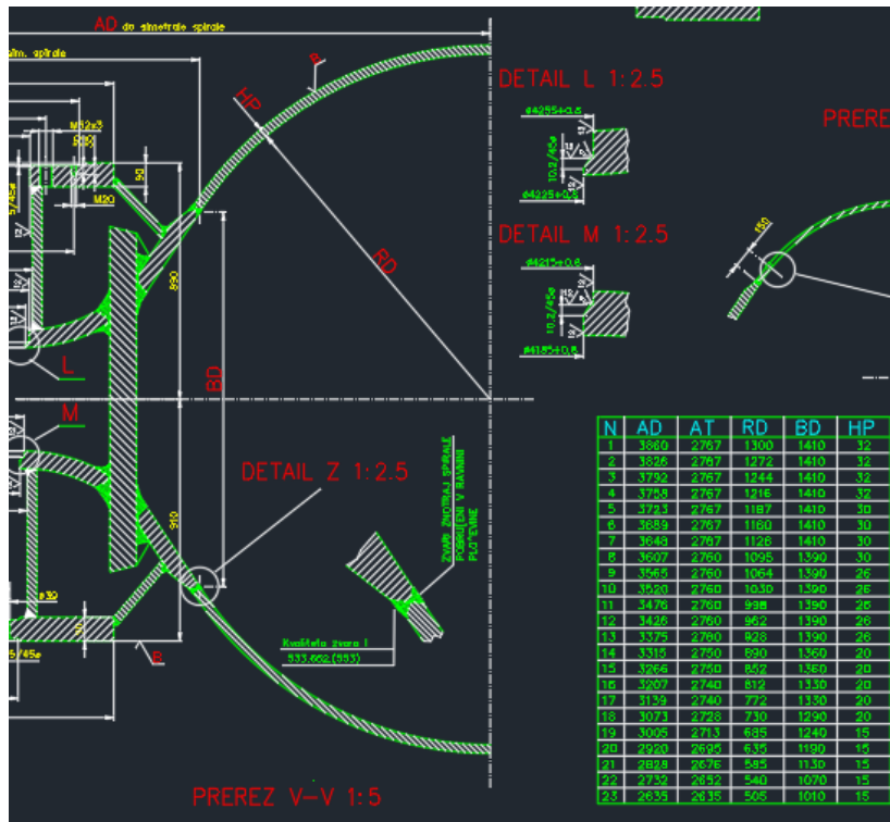
Slika 3-3 Dimenzije charakteristických plocha spirale
