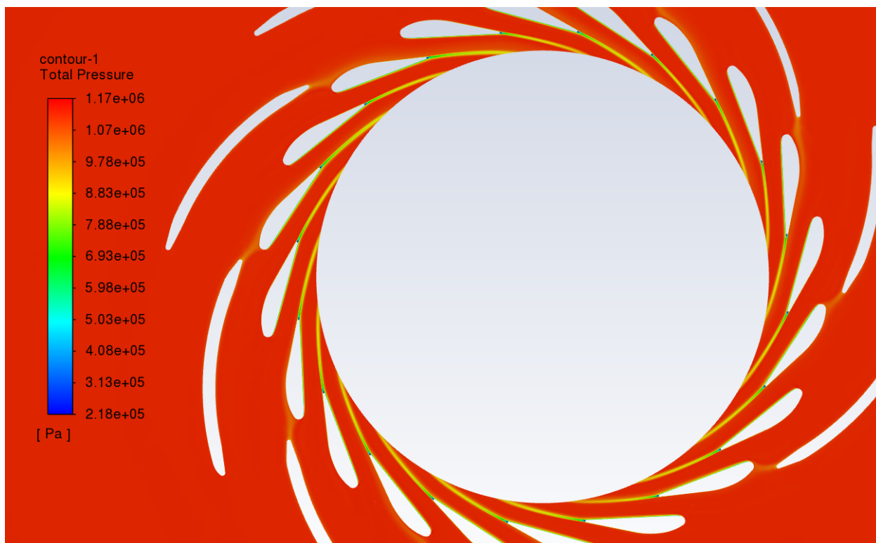
Slika 6-48 Konture totalnog tlaka u iso ravnini
