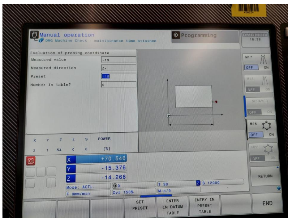
Slika 5.5.: Određivanje nul-točaka
