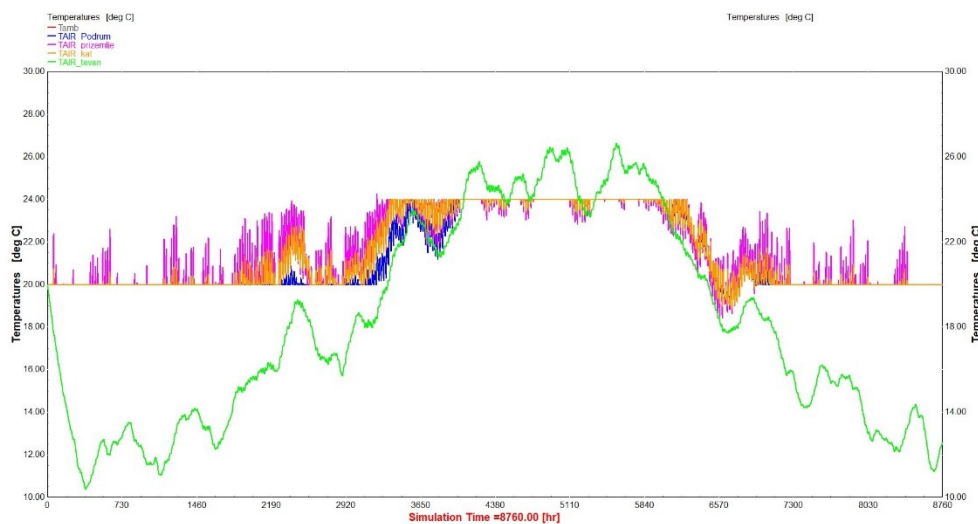
Slika 4.4: raspodjela temperatura tijekom cijele godine za sve etaže modela 1
