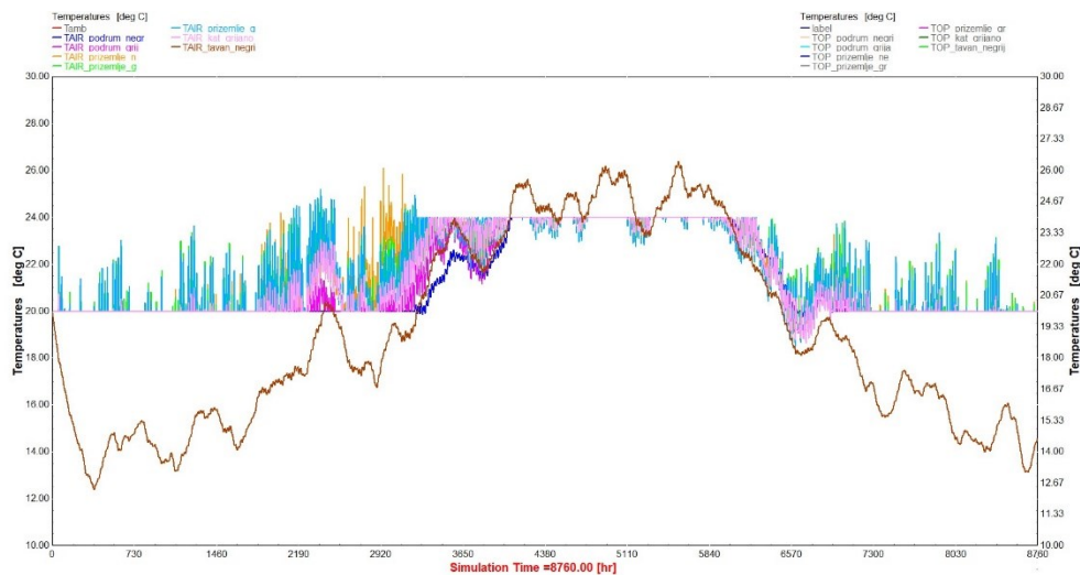
Slika 4.6: raspodjela temperatura tijekom cijele godine za sve zone modela 2
