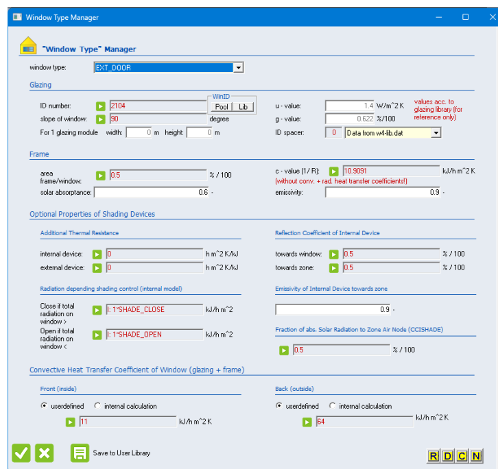
slika 3.6: definiranje otvora na fasadi obiteljske kuće
