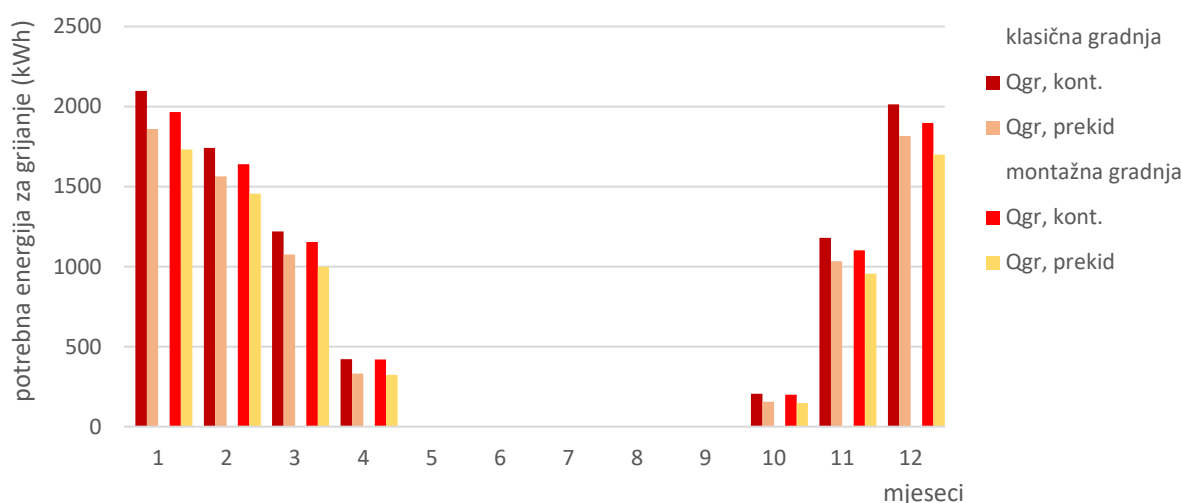
Slika 4.11: usporedni dijagram montažne i klasične gradnje
