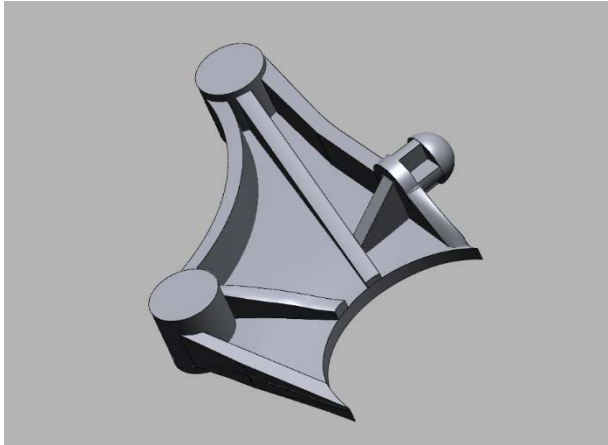
Slika 4.33 Modeliranje ojačanja
