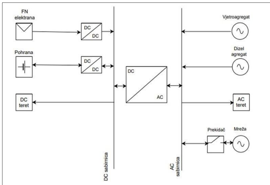
Slika 2.5 Hibridna mikromreža
