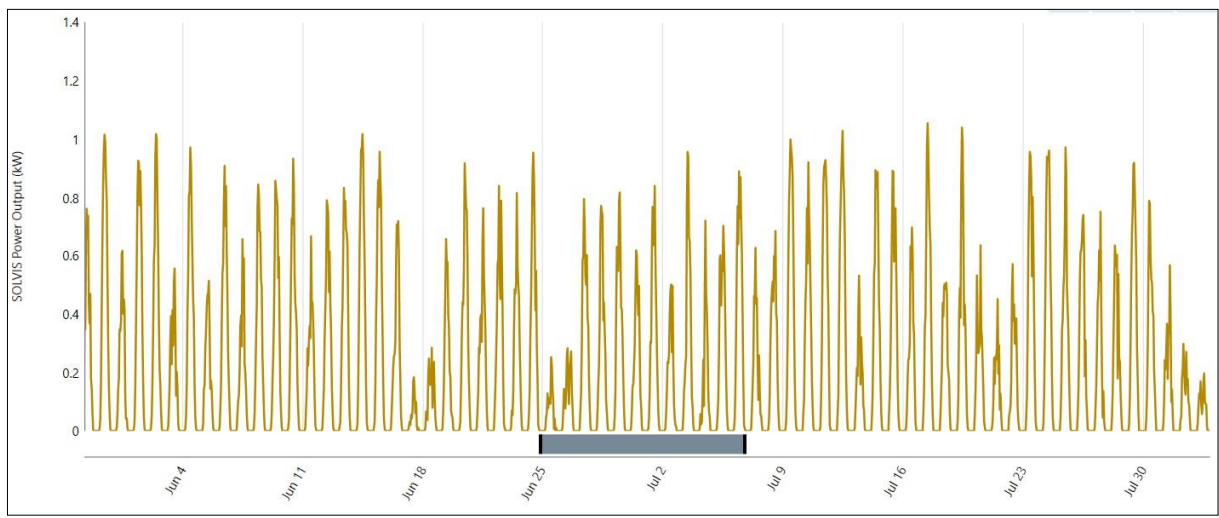
Slika 4.12 Proizvodnja električne energije fotonaponske ćelije za srpanj
