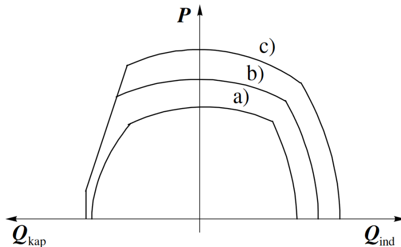
Slika 4.3. Pogonska karta turbogeneratorsa s različitim iznosima pritiska vodika: a) 10^5 Pa; b) 2 \times 10^5 Pa; c) 4 \times 10^5 Pa. [11]
