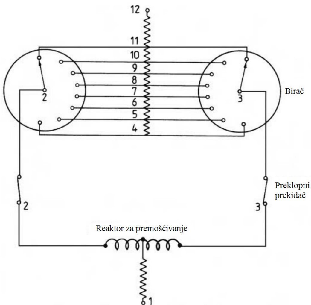
Slika 6.12. Regulacijska sklopka pod opterećenjem s preklopnim prekidačima [13]
