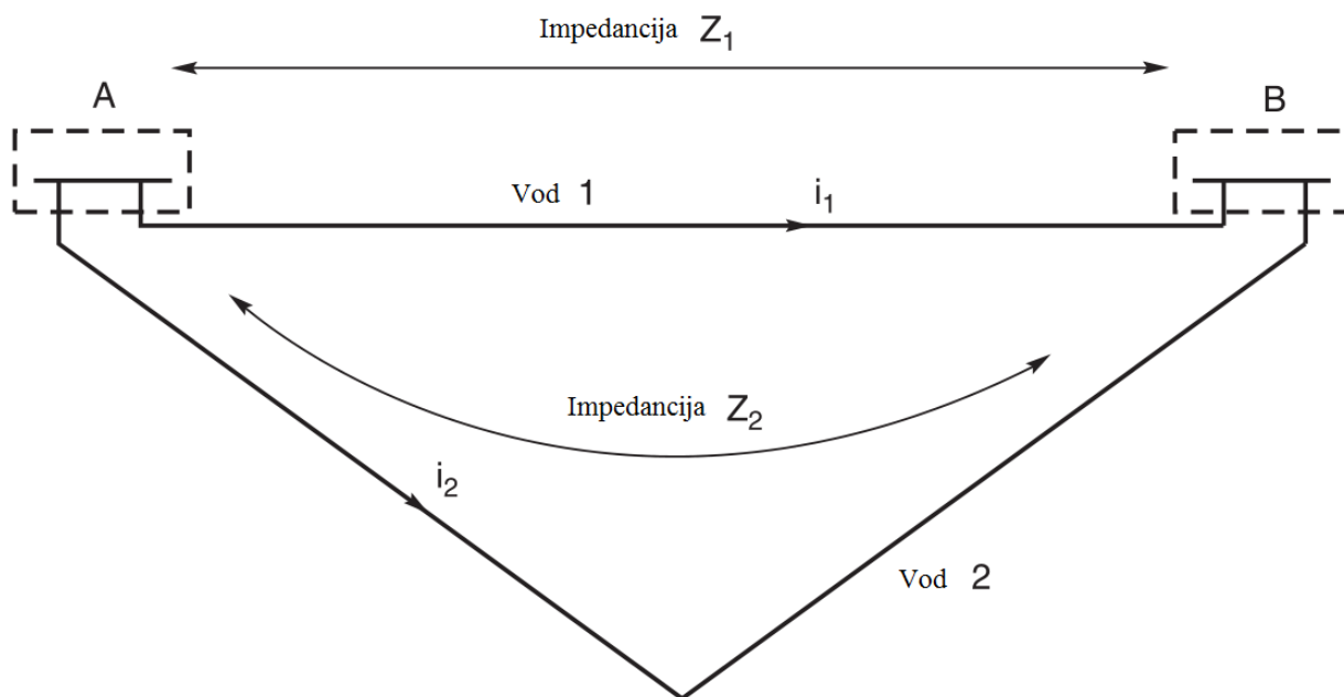
Slika 6.2. Protok struje u mreži određen impedancijama vodova [13]
