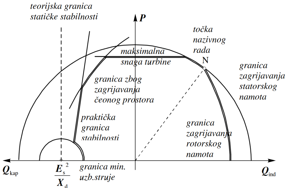
Slika 4.2. Primjer pogonske karte generatora [11]
