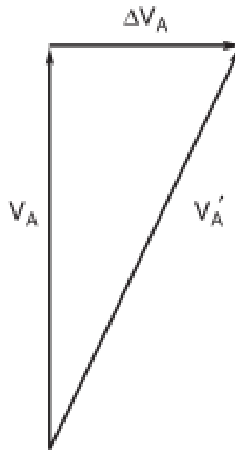
Slika 6.6. Fazorski dijagram jedne faze osnovnog spoja [13]
