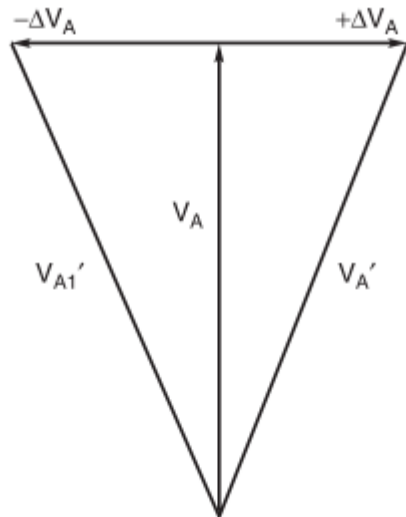
Slika 6.8. Fazorski dijagram funkcionalnog spoja [13]
