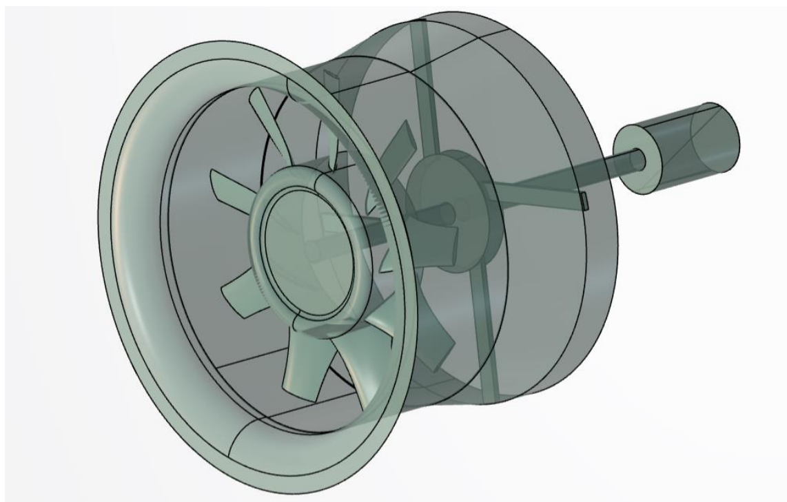
Slika 5.2 Model ventilatora
