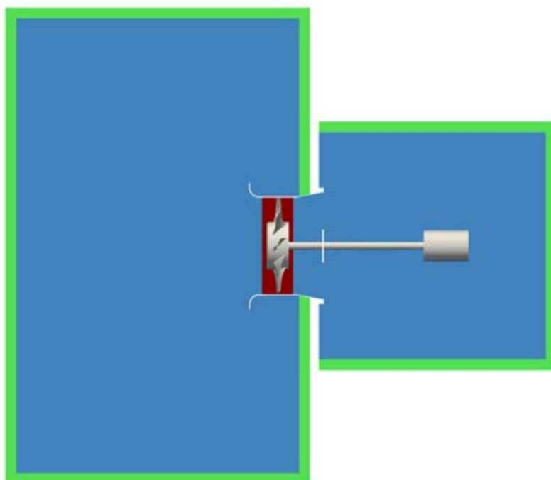
Slika 5.1 Izgled domene za simulaciju akustike [13]
