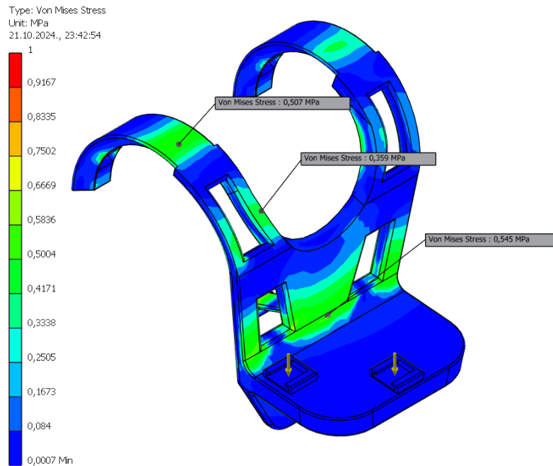
Slika 5.31 Ostala bitnija napreznja prema Von Misesu u cijelom nosaču
