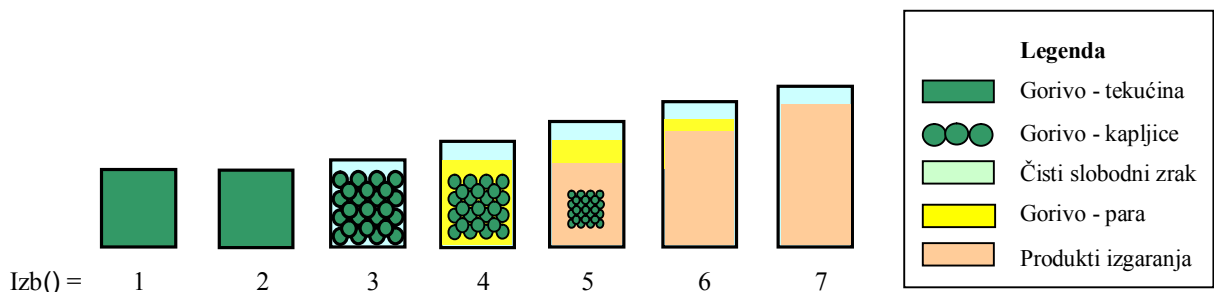
Slika 5.10. Moguća stanja u paketu mlaza goriva
