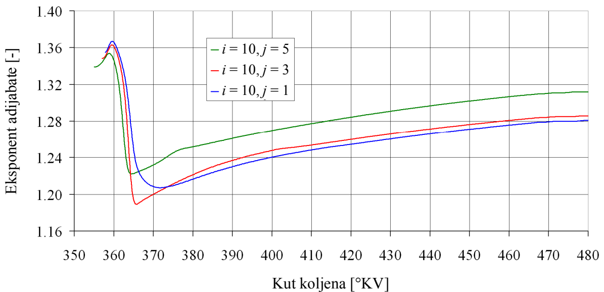
Slika 7.50. Eksponent adijabate za termodinamički volumen paketa mlaza za pakete iz desetoga aksijalnog reda
