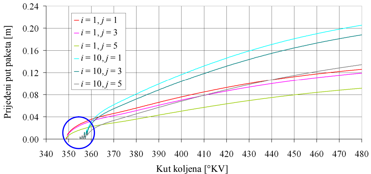
Slika 7.33. Prijeđeni put paketa od mlaznice za različite pakete mlaza
