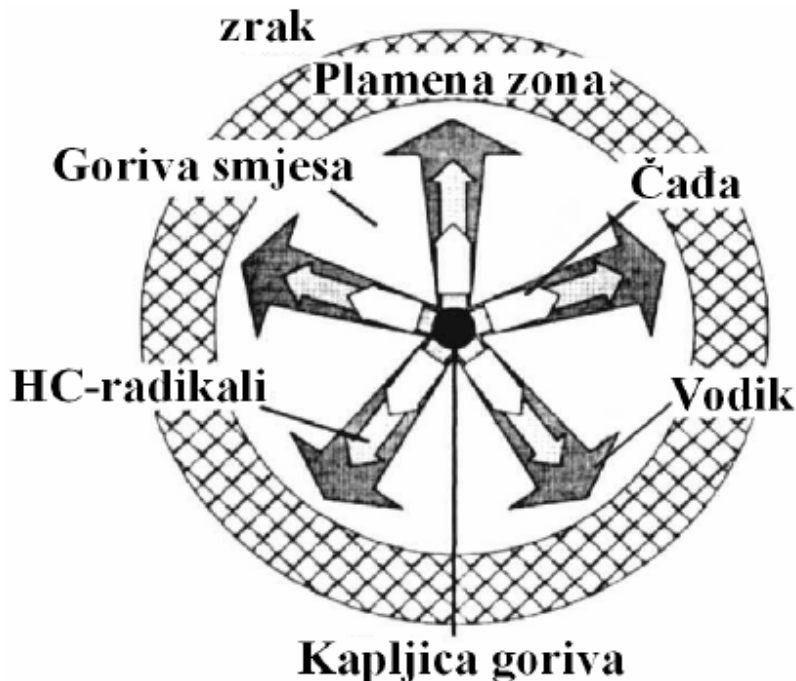
Slika 4.14. Prikaz tvorbe čađe prema difuzijskoj hipotezi [170]
