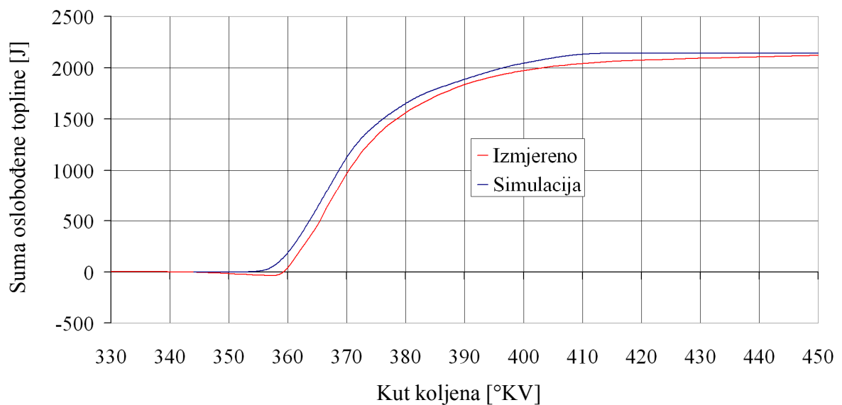
Slika 6.4. Suma oslobodene topline u cilindru za mjernu točku D215HI15
