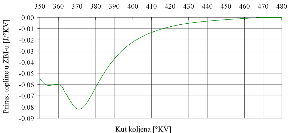
Slika 7.16. Prirast topline u ZBI-u zbog izmjene topline konvekcijom na stijenci
