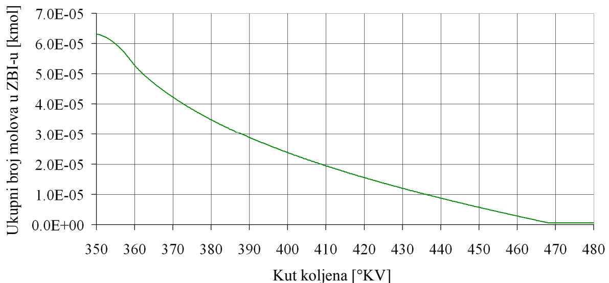
Slika 7.24. Ukupni broj molova u zoni bez izgaranja
