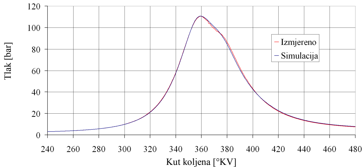
Slika 6.13. Usporedba izmjerenog i izračunatog tlaka u cilindru za mjernu točku D224HI20
